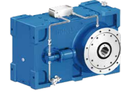
DLZLYJ系列单螺杆挤出机减速机 DLZLYJ Series Gear Units For Single Screw Extruder
